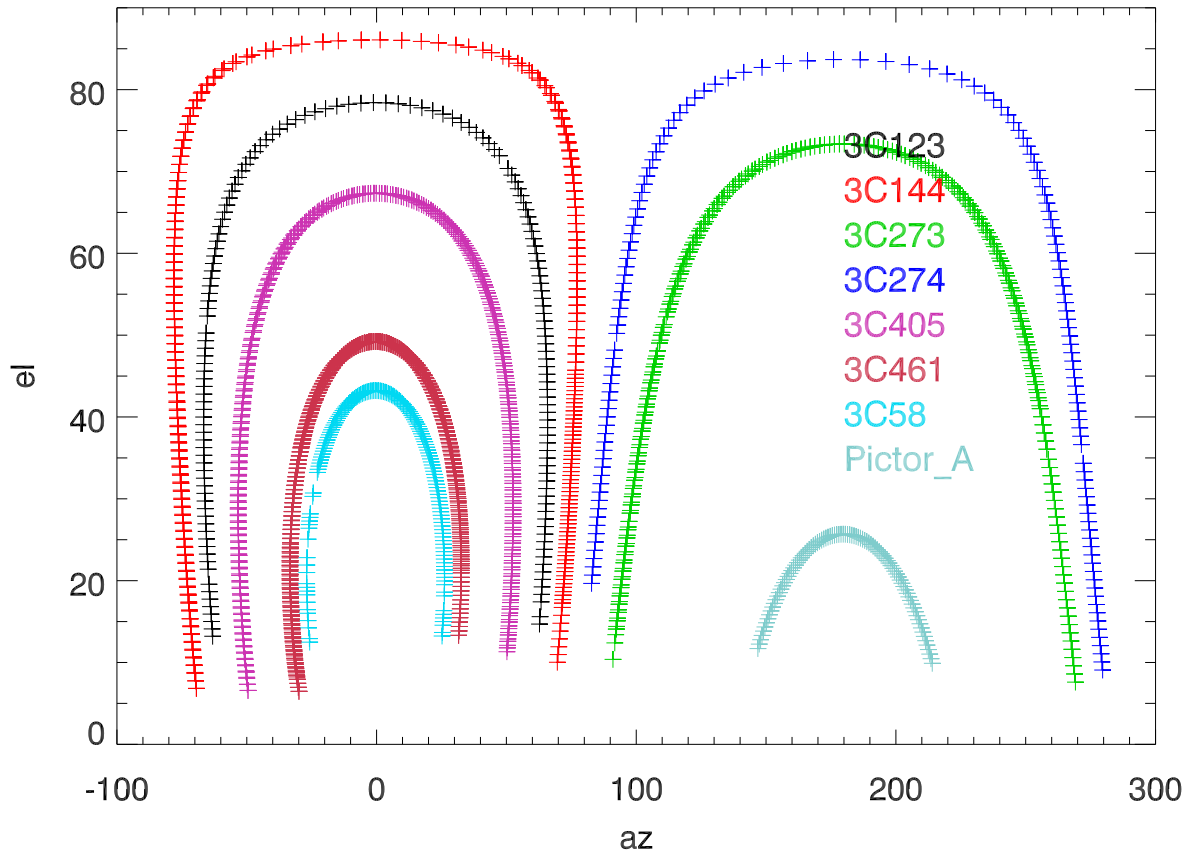
Feb 16 model3A: az el coverage
