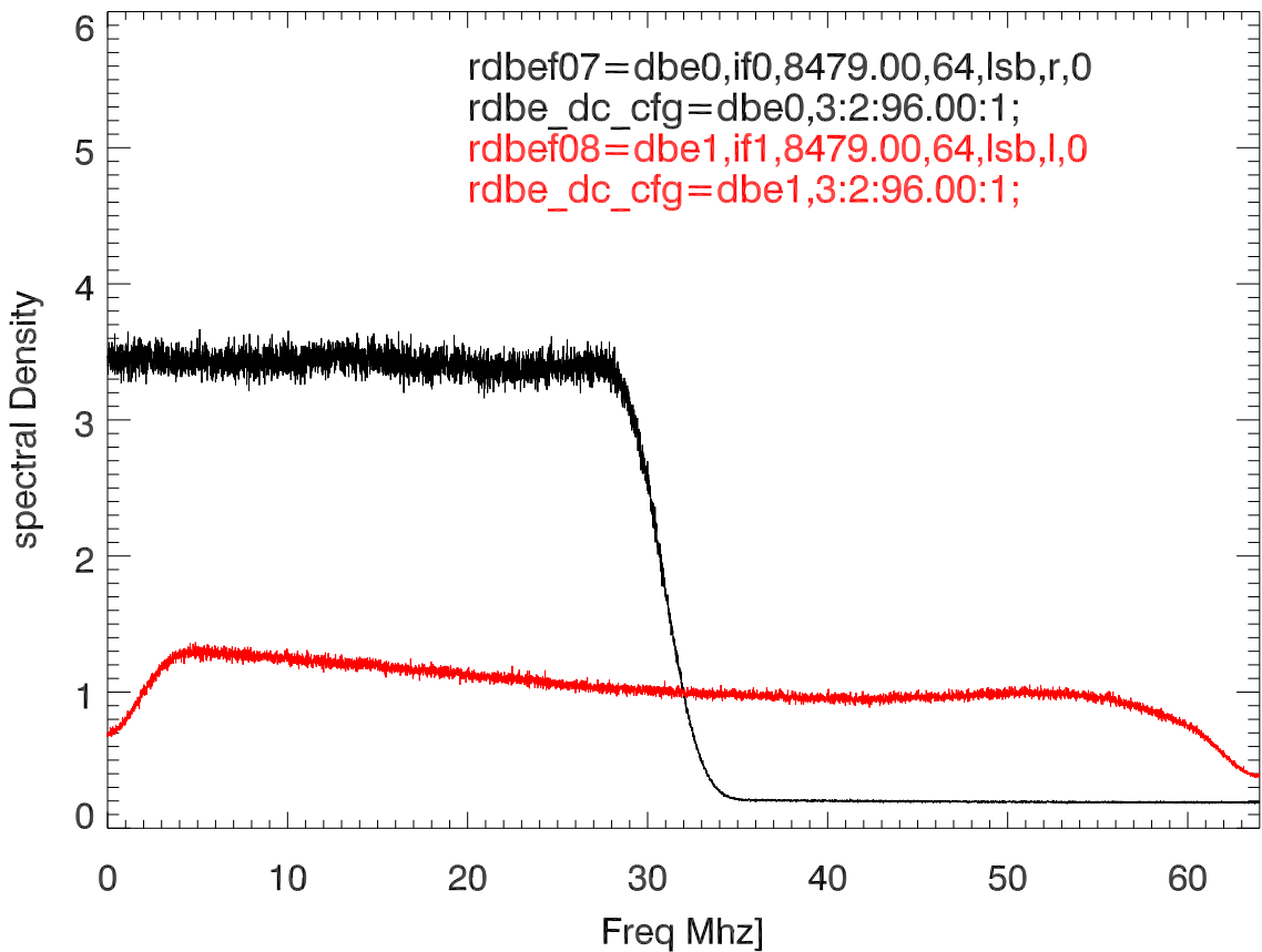
05nov21 fs spectra band:8479
