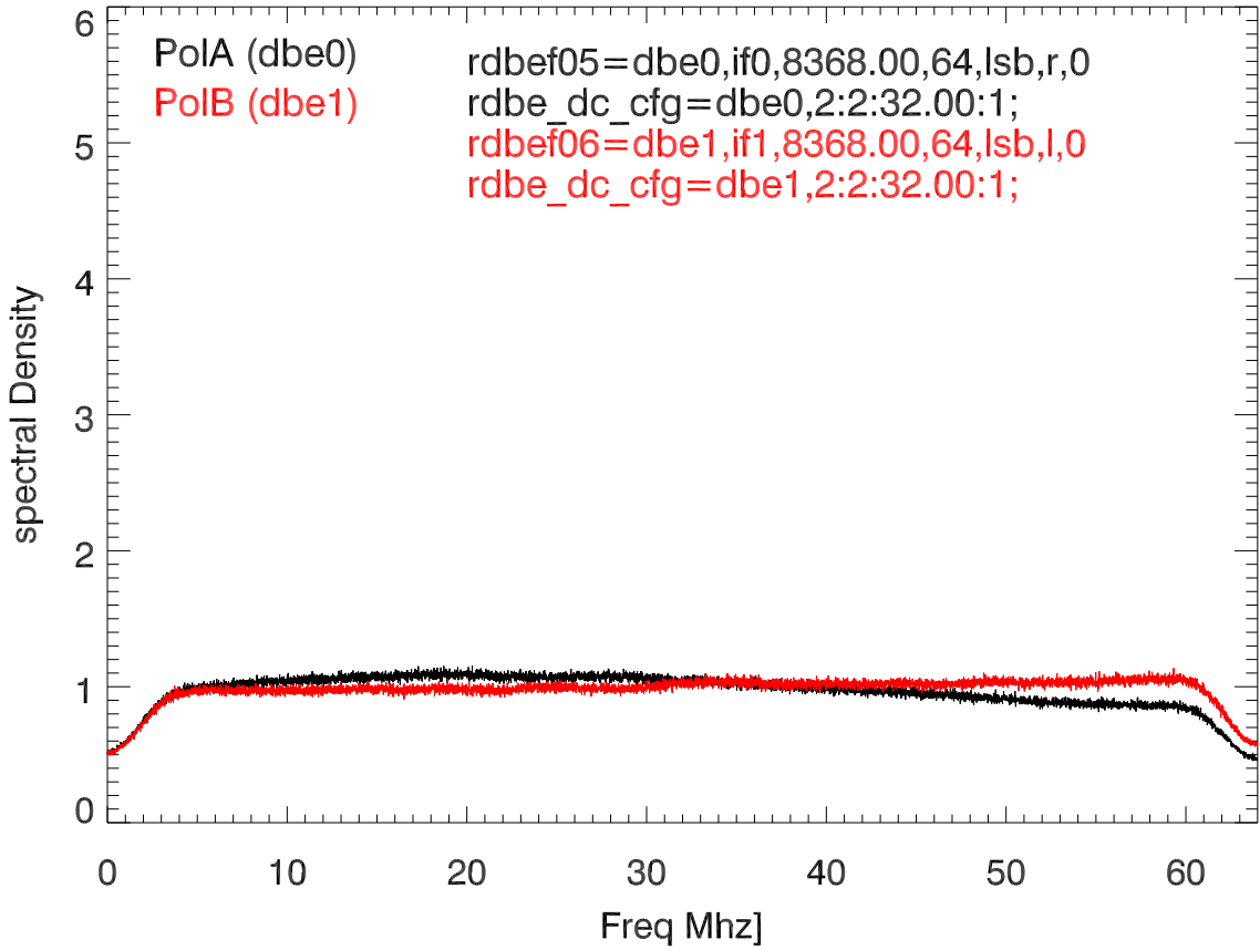
22oct21 fs spectra band:8368
