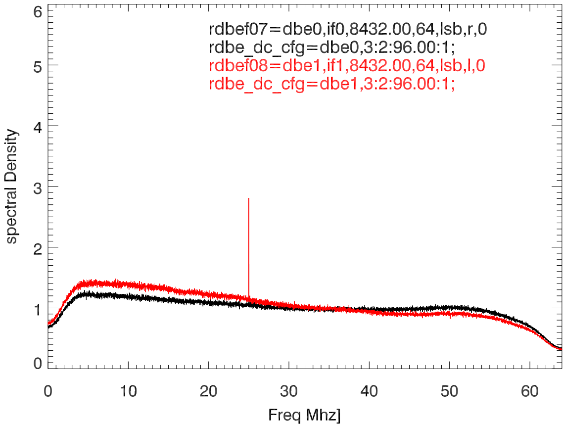
22oct21 fs spectra band:8432
