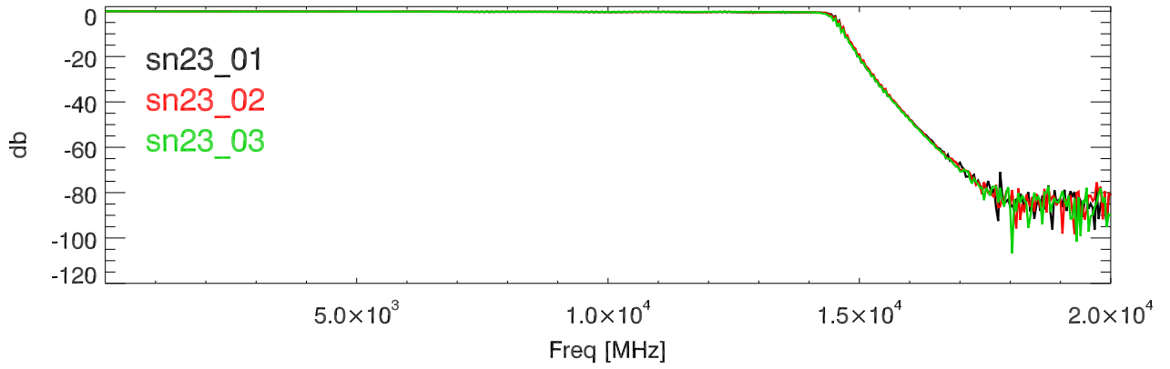
230403: S-parameters for 15GHzg_lowpas. S21
