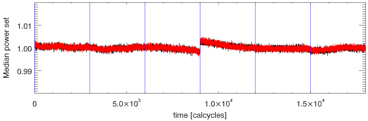
8647 Mhz PoIA
