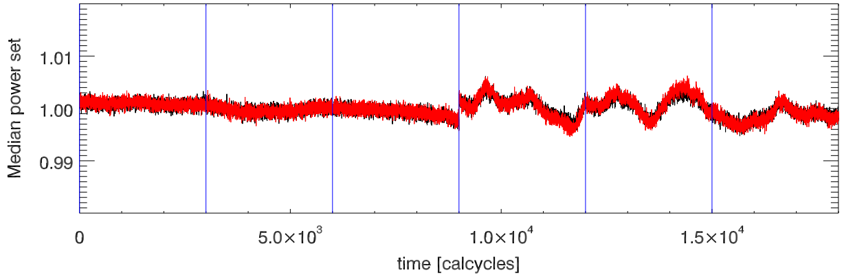
8363 Mhz PoIA
