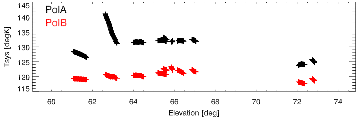
220214 Tsys vs elevation (using 1sec offSrc samples). freqBand:9168
