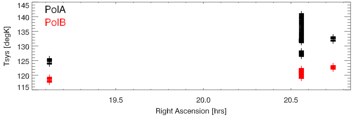
220214 Tsys vs RA (using 1sec offSrc samples). freqBand:9168
