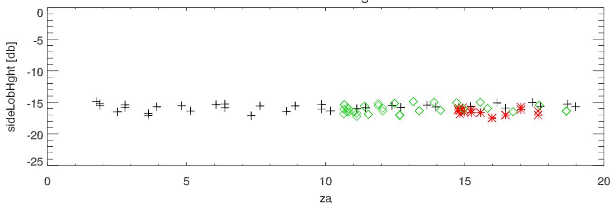
SideLobe Height
