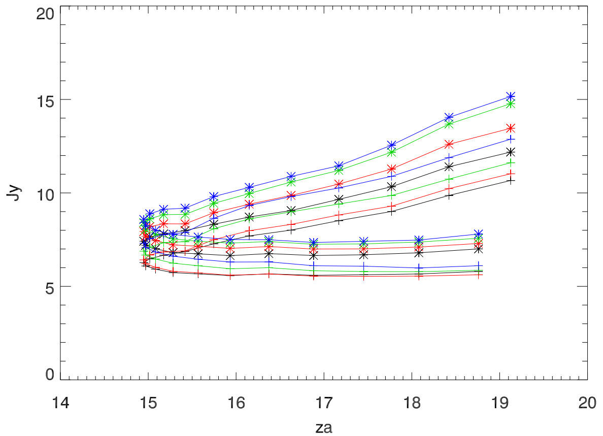
sbh SEFD vs za
