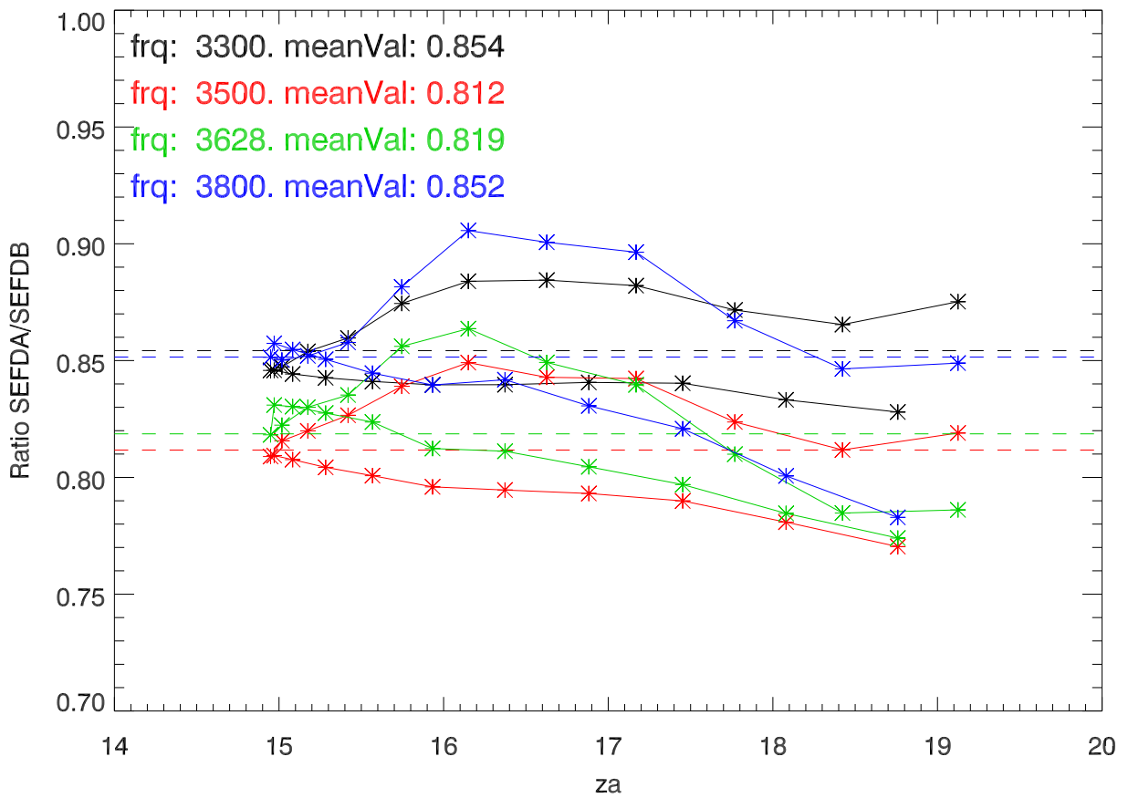
sbh Dec19 SEFDA/SEFDB
