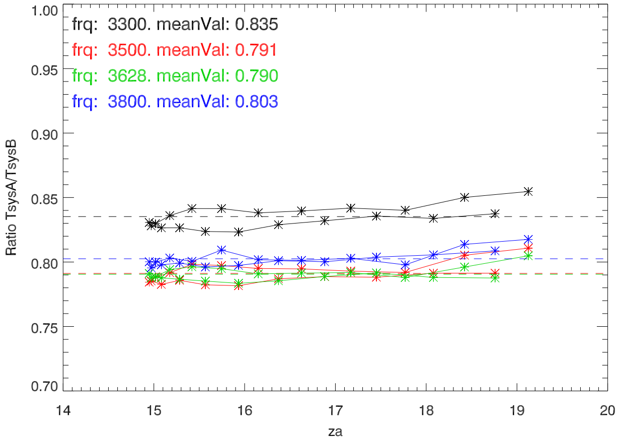
sbh Dec19 TsysA/TsysB
