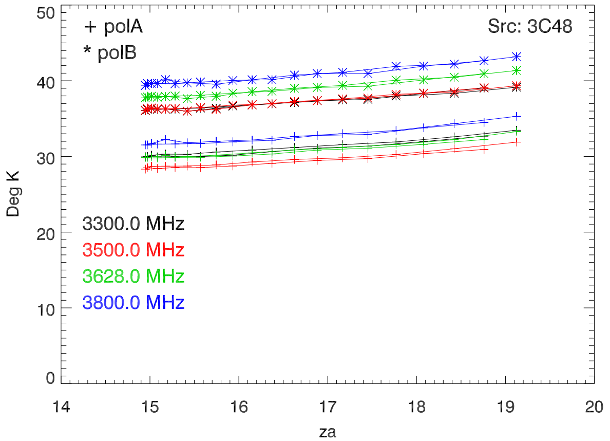
sbh Dec19 x102. Tsys vs za
