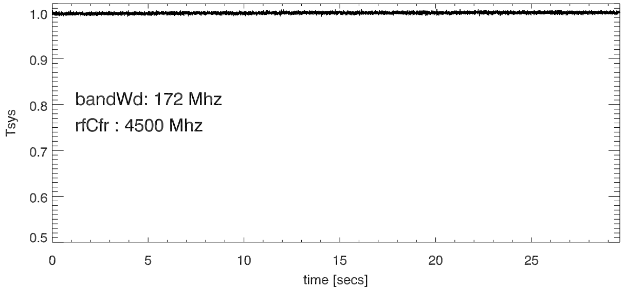
10feb20 cband total power vs time PolA
